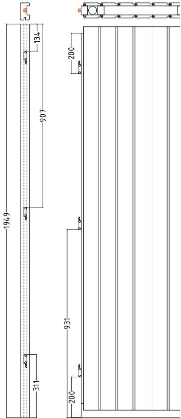
Multiclip
